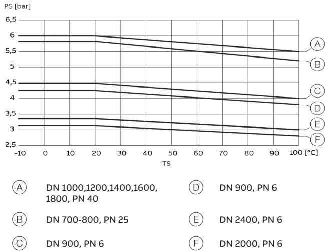
Figure 13 DIN flange, carbon steel, DN 25-600
